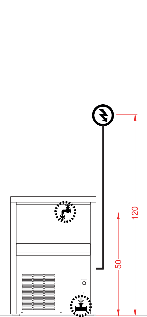
Vista Elevación
