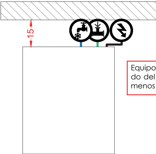
Vista Planta
